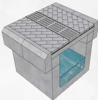
Langkah 6 Memasang Balok Paving Trotoar.
