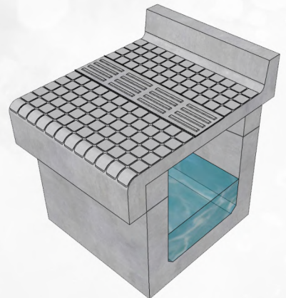
Langkah 3 Penempatan Satria Trotoar Precast.
